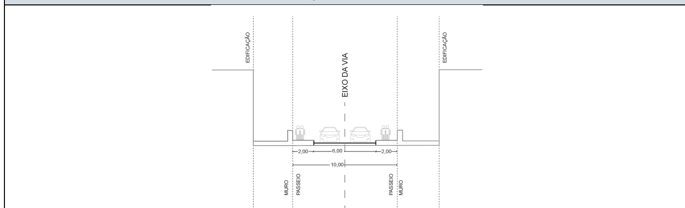
Via 2 – Seção Transversal Planejada (LC nº 482/2014)
