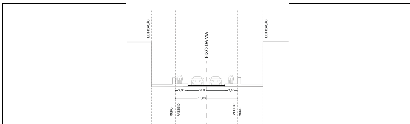
Via 1 – Seção Transversal Planejada (LC nº 482/2014)
