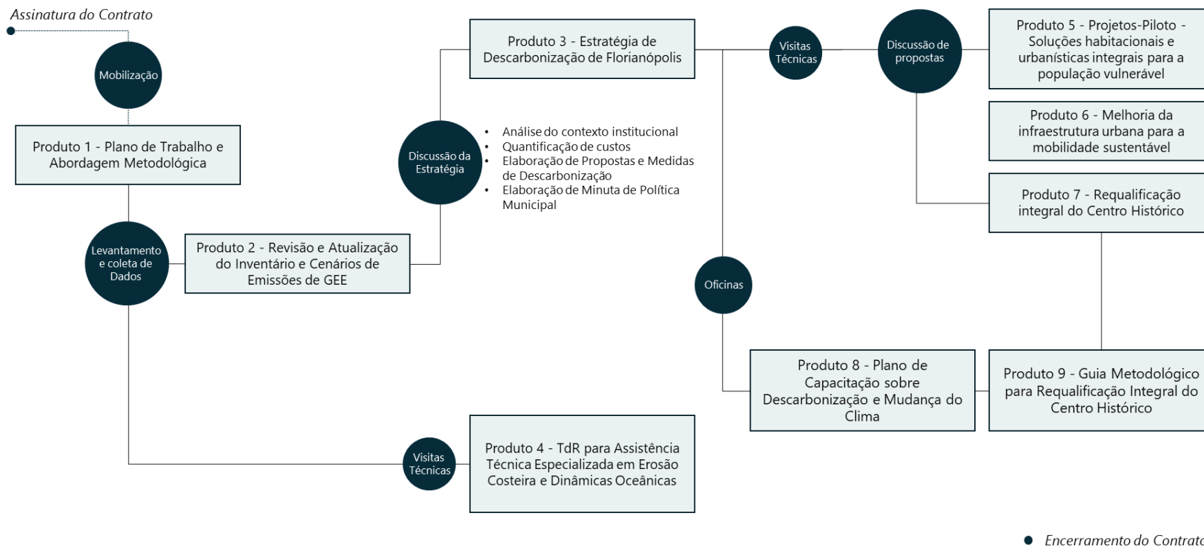
FIGURA 1: ETAPAS METODOLÓGICAS
