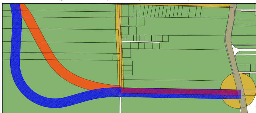
Figura 2 - Alteração do traçado da Via Projetada TR-VP-301
