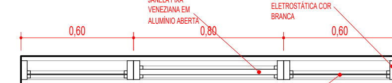
J02 - VISTA PLANTA ESC.: 1:20
