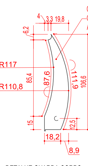
DETALHE GUARDA CORPO PILARETE ESC 1:25
