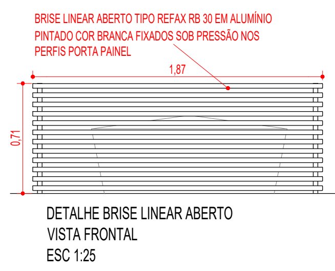
DETALHE BRISE LINEAR ABERTO VISTA FRONTAL ESC 1:25
