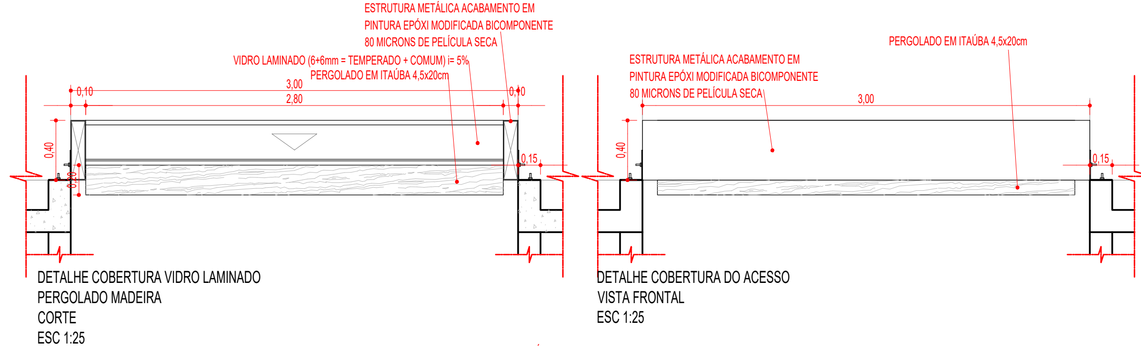
DETALHE COBERTURA DO ACESSO CORTE ESC 1:25
