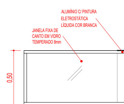
J03 - VISTA ELEVAD. ESC.: 1:20
