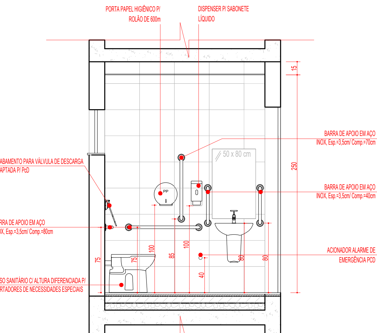
DETALHE SANITÁRIO PNE CORTE ESC 1:25
