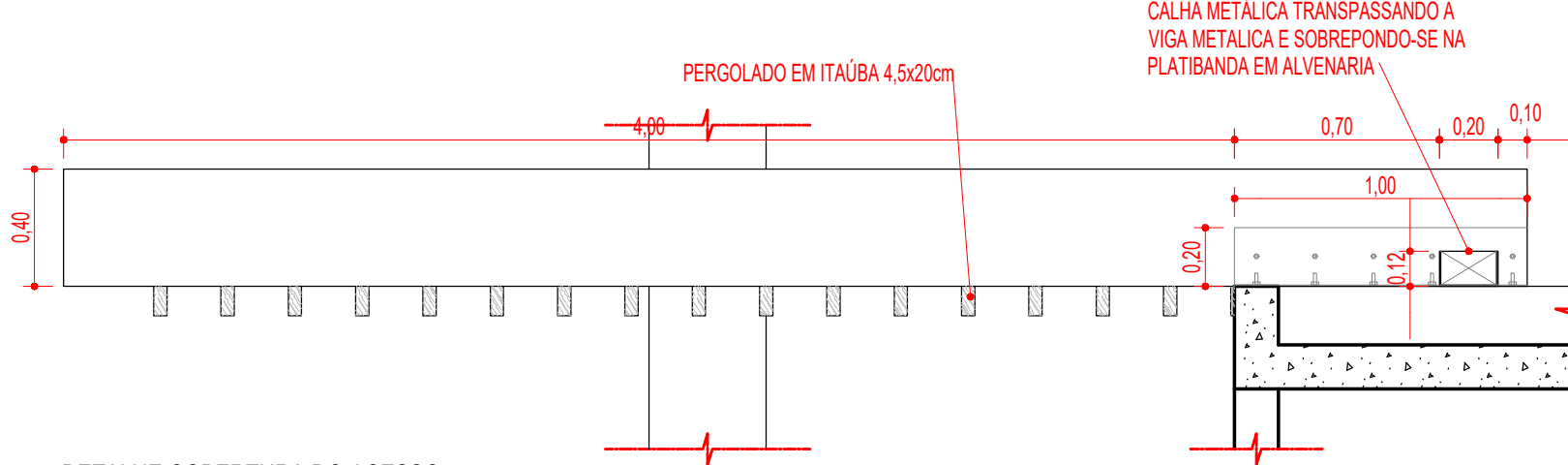
DETALHE COBERTURA DO ACESSO VISTA LATERAL ESC 1:25
