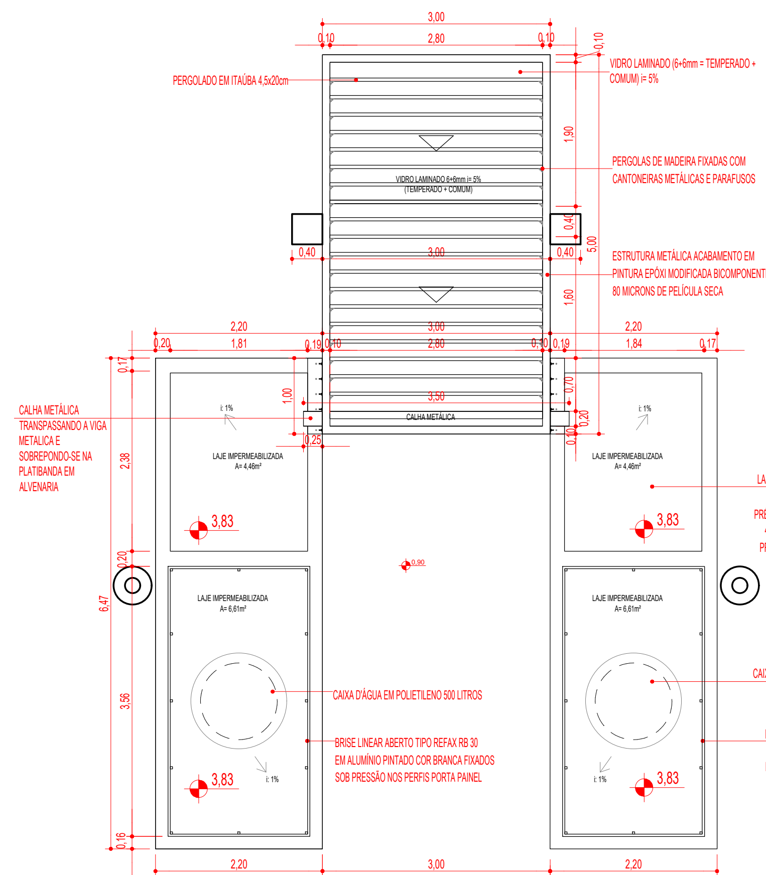
PLANTA BAIXA COBERTURA DO ACESSO / BRISE LINEAR ABERTO VISTA LATERAL ESC 1:50
