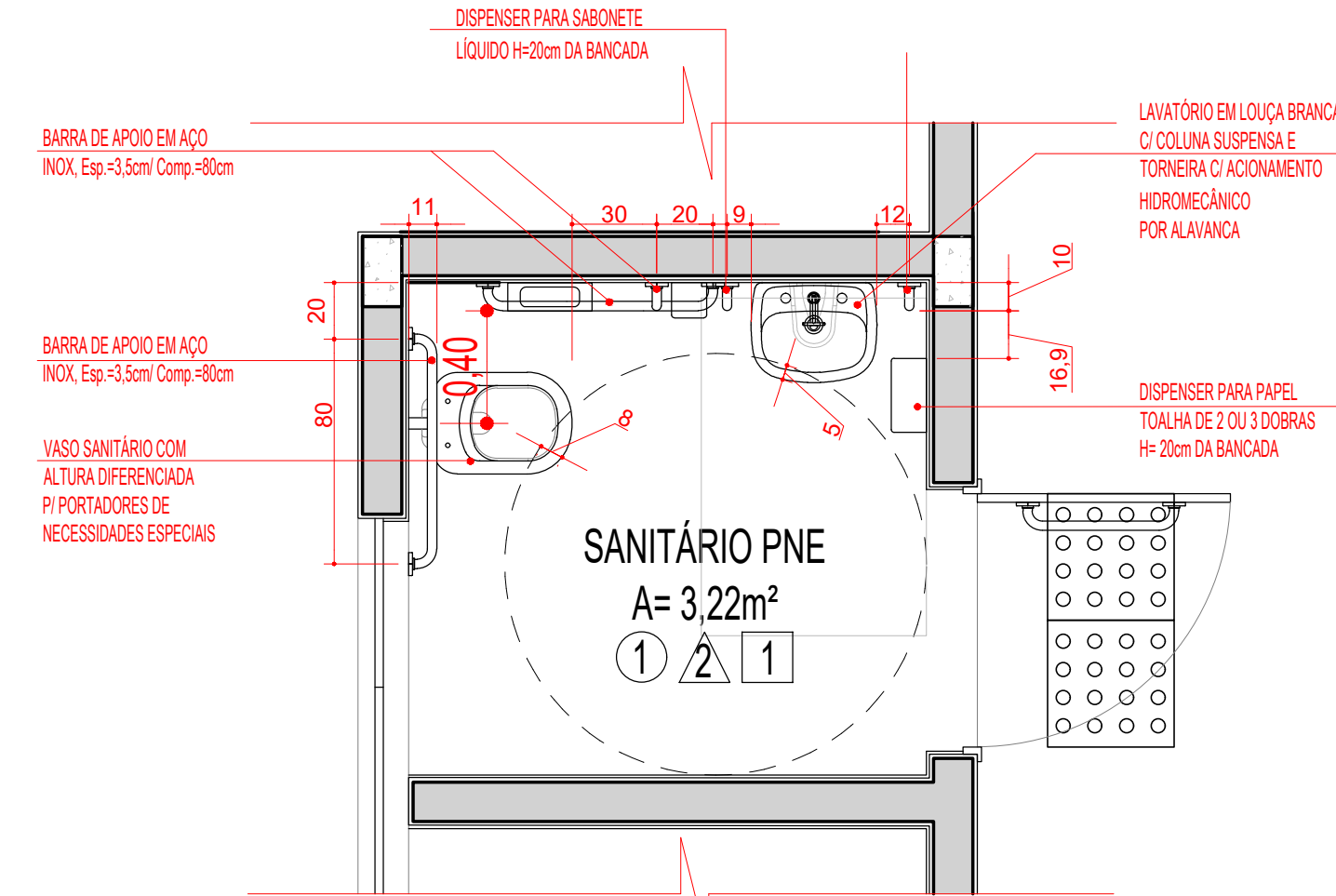
DETALHE SANITÁRIO PNE PLANTA BAIXA ESC 1:25
