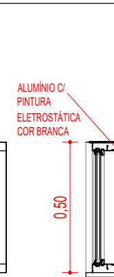
J02 - VISTA CORTE ESC: 1:20
