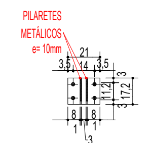
DETALHE GUARDA CORPO CHAPA DE APOIO ESC 1:25
