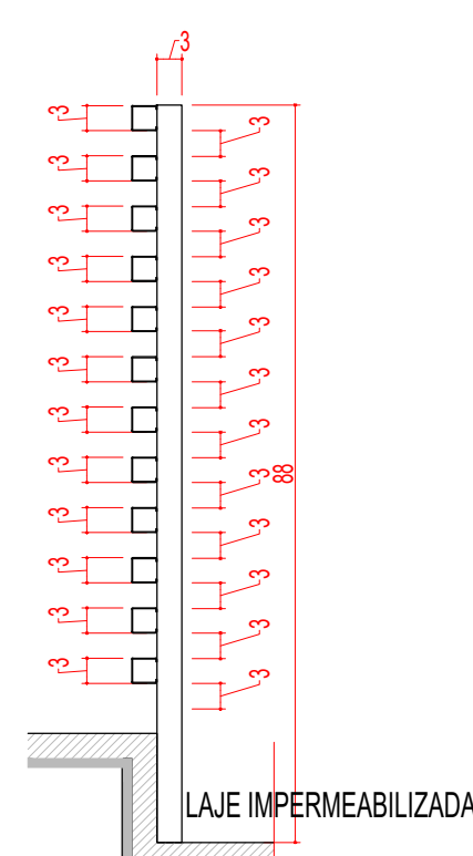
DETALHE BRISE LINEAR ABERTO ESC 1:10
