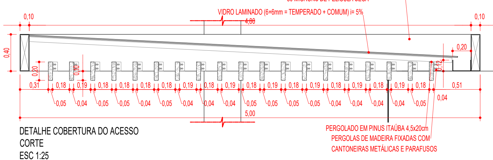
DETALHE COBERTURA DO ACESSO CORTE ESC 1:25
