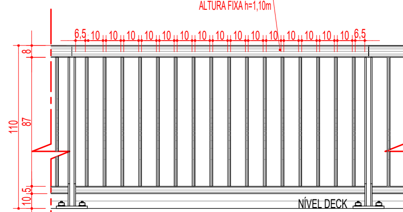
VISTA EXTERNA - GUARDA CORPO ESC 1:25
