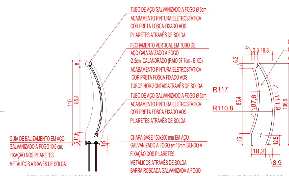
DETALHE GUARDA CORPO FECHAMENTO ESC 1:25
