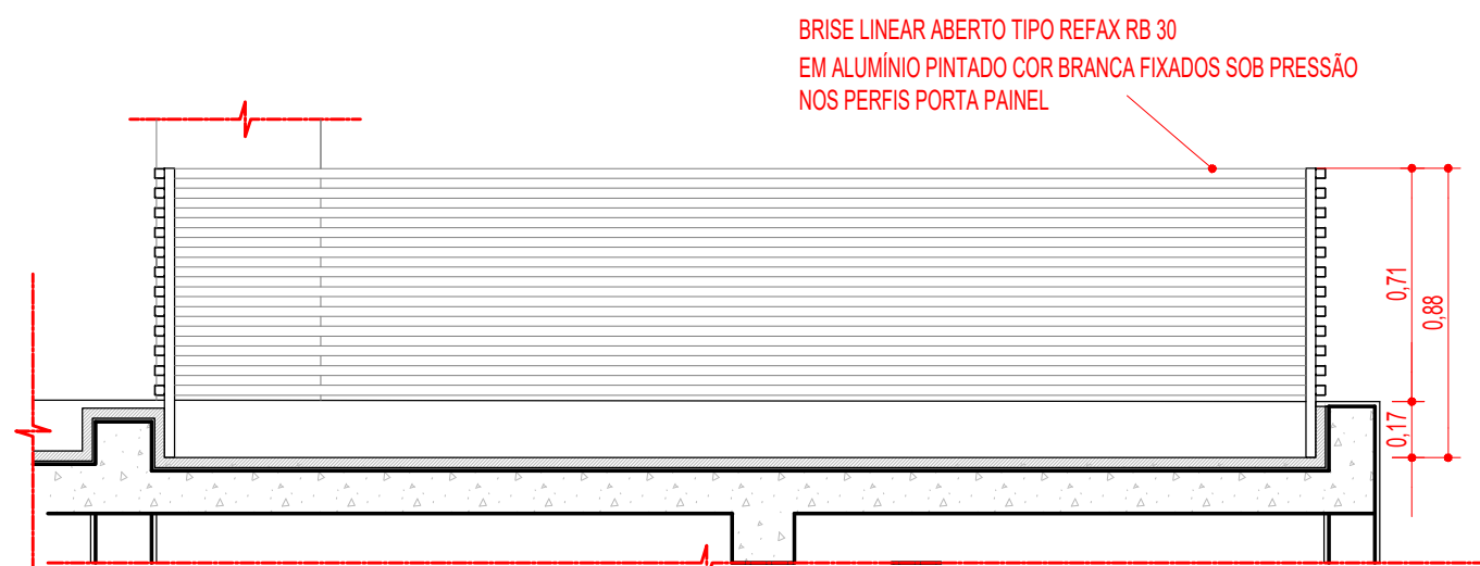
DETALHE BRISE LINEAR ABERTO CORTE LATERAL ESC 1:25
